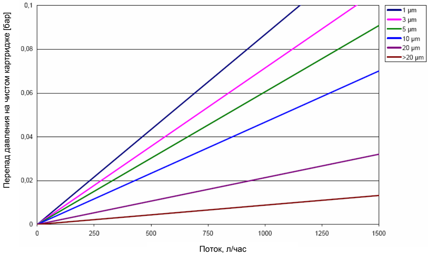
Поток через 10" amaPure HS картридж
