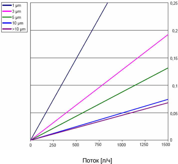
Поток воды л/ч через 10" картридж amaTech UE/PW
