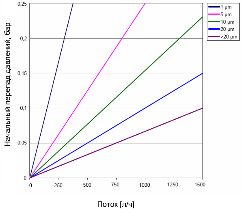
Поток воды л/ч через 10" картридж amaTech CE
